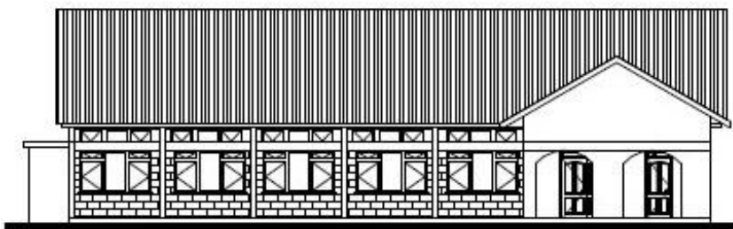
Zuidaanzicht Social Hall Kiriita/Kapsara.
